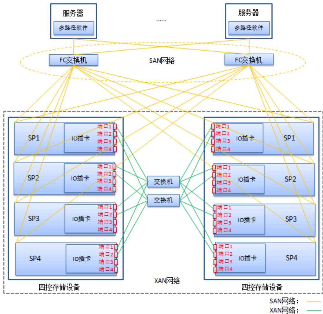
图4-4 四控 XAN 典型组网图（交换机连接）
